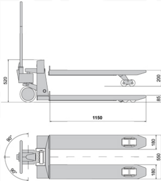
Dimensioni transpallet in mm
