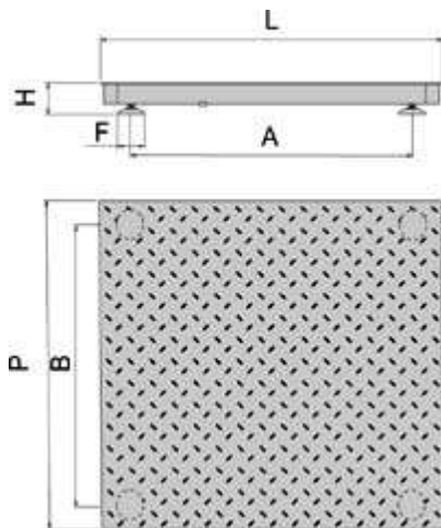
Piattaforme elettroniche di pesatura serie EL.
